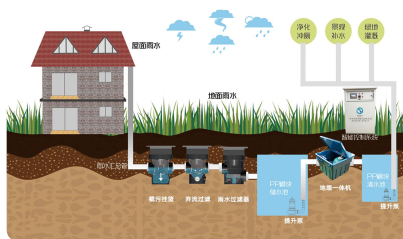
5.3.2雨水回收利用技术
